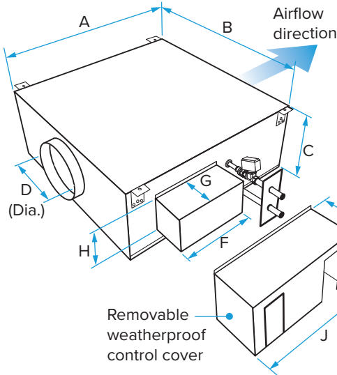
SUPPLY FAN SIZE DS2H - DATA LPHW 82/71 (°C)
