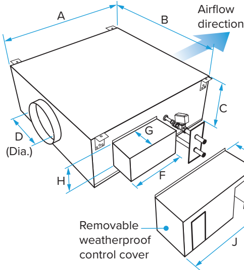
SUPPLY FAN SIZE DS7 - DATA LPHW 82/71 (°C)
