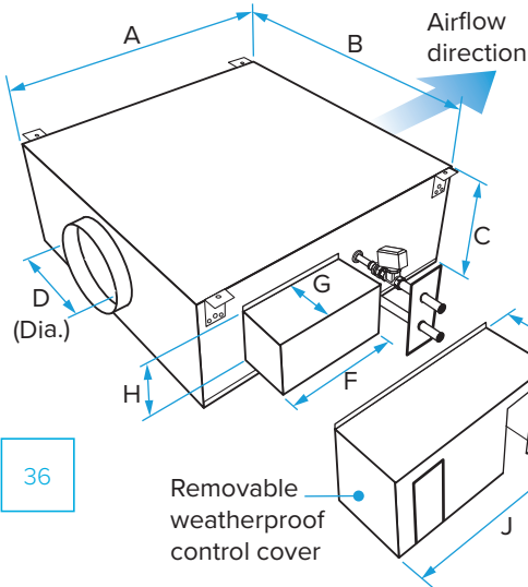
SUPPLY FAN SIZE DS4H - DATA LPHW 82/71 (°C)
