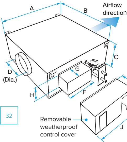
SUPPLY FAN SIZE DS2 - DATA LPHW 82/71 (°C)
