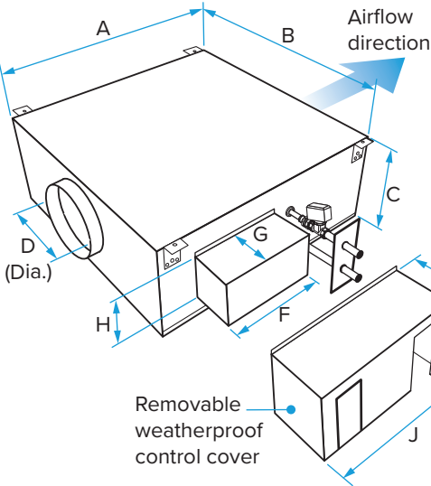
SUPPLY FAN SIZE DS5 - DATA LPHW 82/71 (°C)
