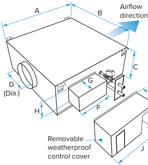
SUPPLY FAN SIZE DS4 - DATA LPHW 82/71 (°C)
